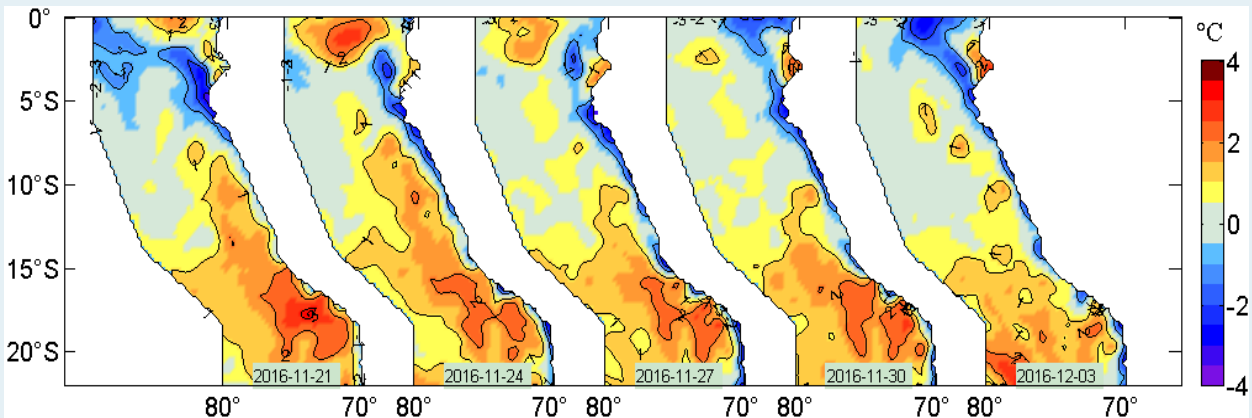
Figura 2. Anomalías de la temperatura superficial del agua (°C) en el mar peruano, cada tres días, entre el 21 de noviembre y 03 de diciembre del 2016. Datos: AVHRR Global Reyn_SmithOiv2R (Reynolds, et. al., 2007) de CMB/EMC/NCEP de la NOAA. Procesamiento: IMARPE.
