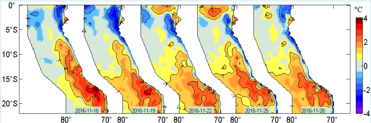
Figura 2. Anomalías de la temperatura superficial del agua (°C) en el mar peruano, cada tres días, entre el 16 y 28 de noviembre del 2016. Datos: AVHRR Global Reyn_SmithOiv2R (Reynolds, et. al., 2007) de CMB/EMC/NCEP de la NOAA. Procesamiento: IMARPE.
