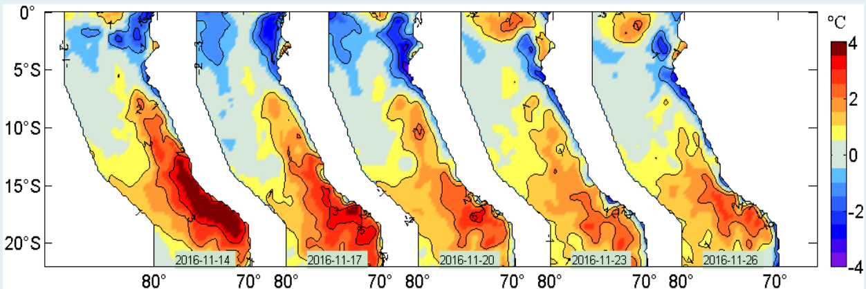
Figura 2. Anomalías de la temperatura superficial del agua (°C) en el mar peruano, cada tres días, entre el 14 y 26 de noviembre del 2016. Datos: AVHRR Global Reyn_SmithOiv2R (Reynolds, et. al., 2007) de CMB/EMC/NCEP de la NOAA. Procesamiento: IMARPE.
