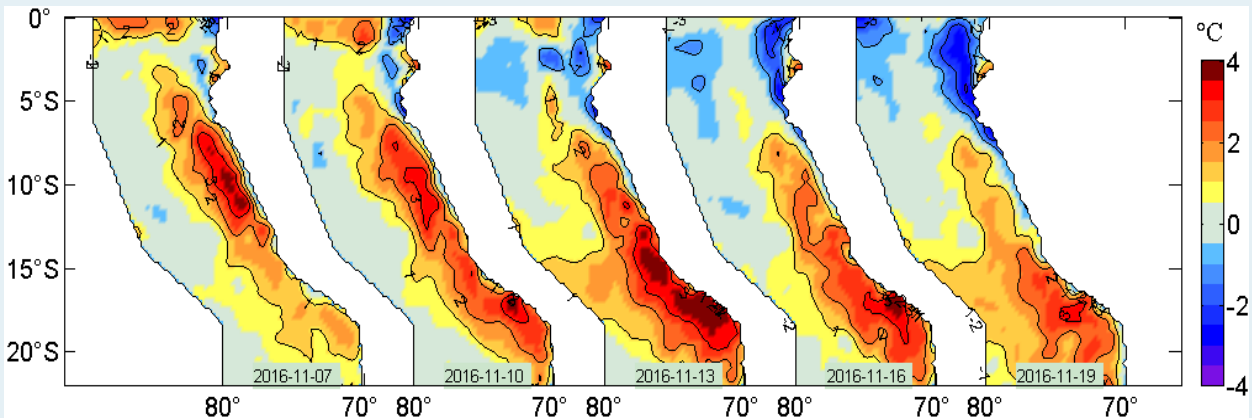
Figura 2. Anomalías de la temperatura superficial del agua (°C) en el mar peruano, cada tres días, entre el 07 y 19 de noviembre del 2016. Datos: AVHRR Global Reyn_SmithOIv2R (Reynolds, et. al., 2007) de CMB/EMC/NCEP de la NOAA. Procesamiento: IMARPE.
