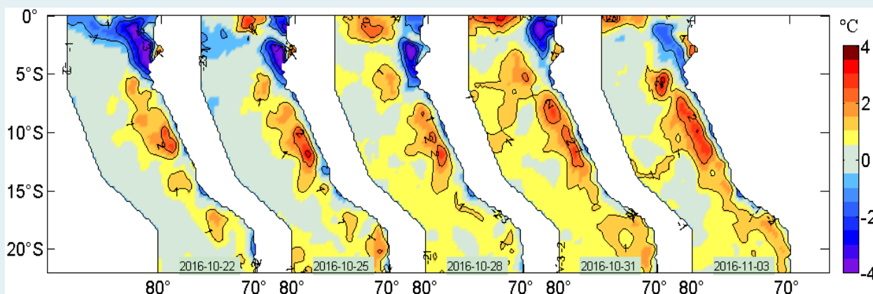
Figura 2. Anomalías de la temperatura superficial del agua (°C) en el mar peruano, cada tres días, entre el 22 de octubre y 03 de noviembre del 2016. Datos: AVHRR Global Reyn_SmithOiv2R (Reynolds, et. al., 2007) de CMB/EMC/NCEP de la NOAA. Procesamiento: IMARPE.
