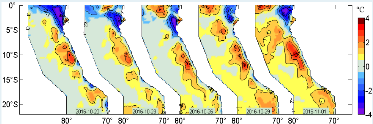
Figura 2. Anomalías de la temperatura superficial del agua (°C) en el mar peruano, cada tres días, entre el 20 de octubre y 01 de noviembre del 2016. Datos: AVHRR Global Reyn_SmithOiv2R (Reynolds, et. al., 2007) de CMB/EMC/NCEP de la NOAA. Procesamiento: IMARPE.
