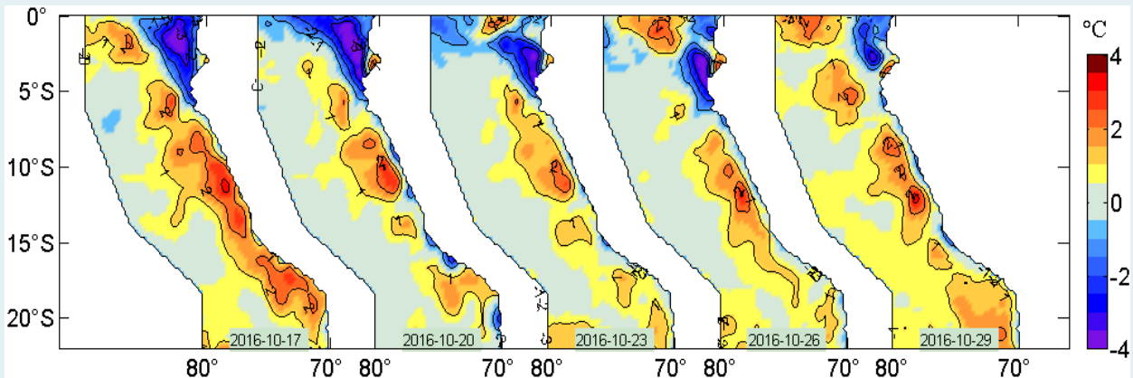
Figura 2. Anomalías de la temperatura superficial del agua (°C) en el mar peruano, cada tres días, entre el 17 y 29 de octubre del 2016. Datos: AVHRR Global Reyn_SmithOiv2R (Reynolds, et. al., 2007) de CMB/EMC/NCEP de la NOAA. Procesamiento: IMARPE.
