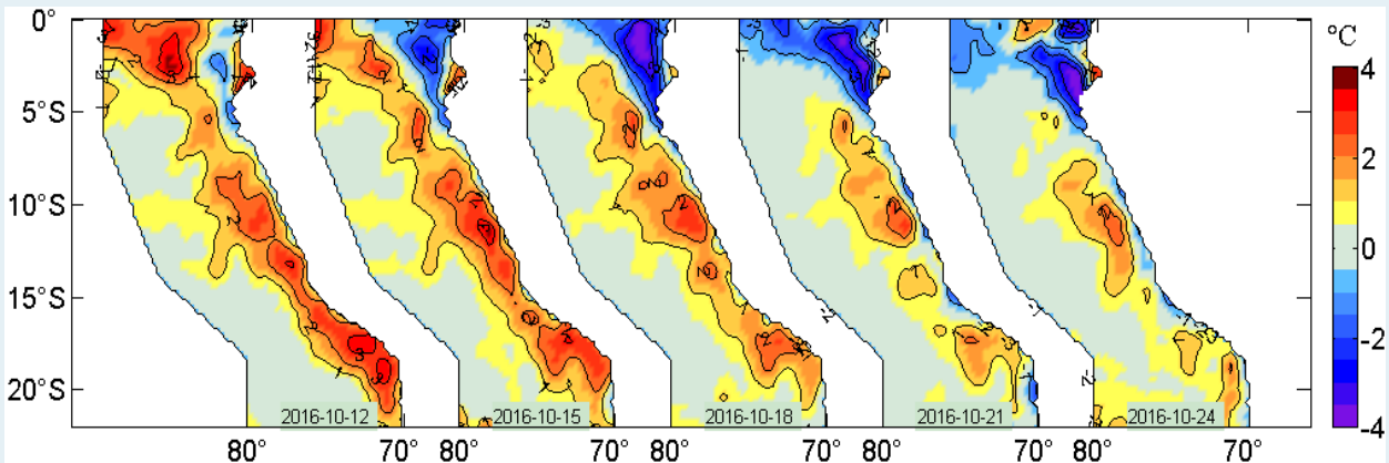
Figura 2. Anomalías de la temperatura superficial del agua (°C) en el mar peruano, cada tres días, entre el 12 y 24 de octubre del 2016. Datos: AVHRR Global Reyn_SmithOlv2R (Reynolds, et. al., 2007) de CMB/EMC/NCEP de la NOAA. Procesamiento: IMARPE.
