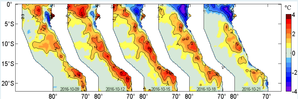
Figura 2. Anomalías de la temperatura superficial del agua (°C) en el mar peruano, cada tres días, entre el 09 y 21 de octubre del 2016. Datos: AVHRR Global Reyn_SmithOiv2R (Reynolds, et. al., 2007) de CMB/EMC/NCEP de la NOAA. Procesamiento: IMARPE.
