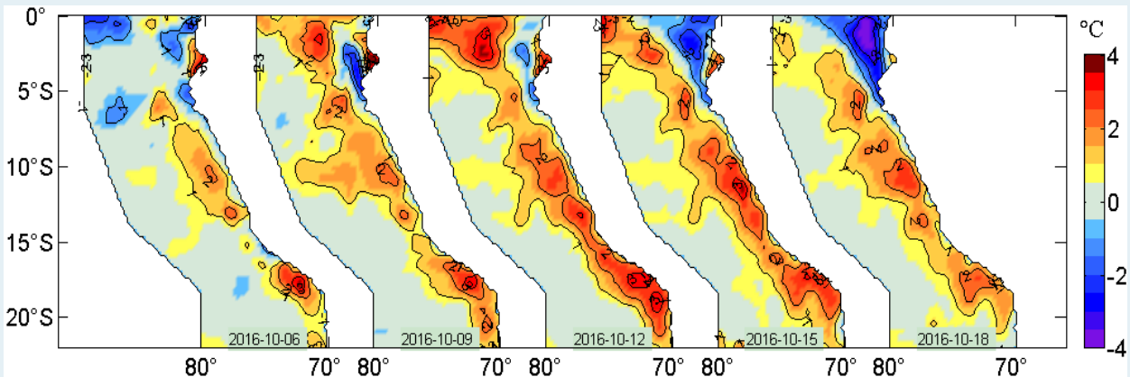
Figura 2. Anomalías de la temperatura superficial del agua (°C) en el mar peruano, cada tres días, entre el 06 y 18 de octubre del 2016. Datos: AVHRR Global Reyn_SmithOiv2R (Reynolds, et. al., 2007) de CMB/EMC/NCEP de la NOAA. Procesamiento: IMARPE.
