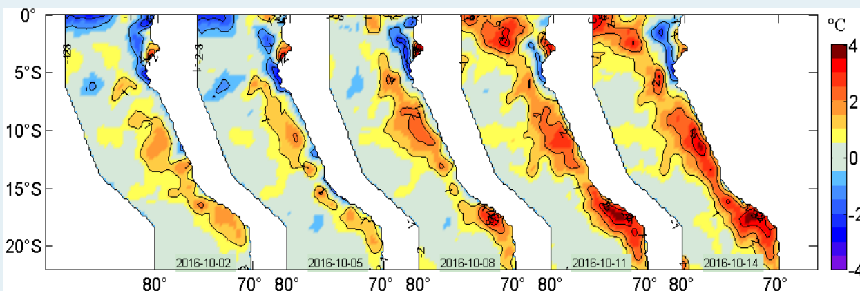
Figura 2. Anomalías de la temperatura superficial del agua (°C) en el mar peruano, cada tres días, entre el 02 y 14 de octubre del 2016. Datos: AVHRR Global Reyn_SmithOIv2R (Reynolds, et. al., 2007) de CMB/EMC/NCEP de la NOAA. Procesamiento: IMARPE.
