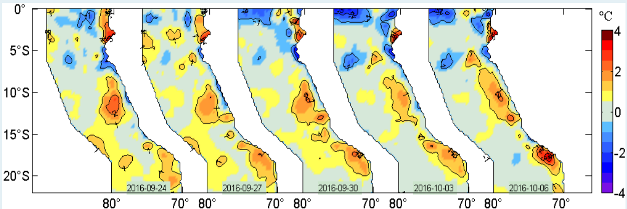
Figura 2. Anomalías de la temperatura superficial del agua (°C) en el mar peruano, cada tres días, entre el 24 de setiembre y 06 de octubre del 2016. Datos: AVHRR Global Reyn_SmithOiv2R (Reynolds, et. al., 2007) de CMB/EMC/NCEP de la NOAA. Procesamiento: IMARPE.
