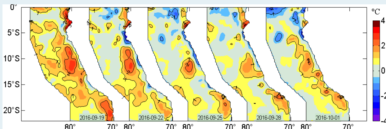
Figura 2. Anomalías de la temperatura superficial del agua (°C) en el mar peruano, cada tres días, entre el 19 de setiembre y 01 de octubre del 2016. Datos: AVHRR Global Reyn_SmithOlv2R (Reynolds, et. al., 2007) de CMB/EMC/NCEP de la NOAA. Procesamiento: IMARPE.
