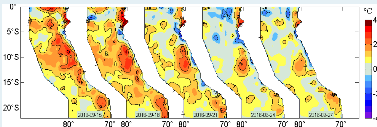
Figura 2. Anomalías de la temperatura superficial del agua (°C) en el mar peruano, cada tres días, entre el 15 y 27 de setiembre del 2016. Datos: AVHRR Global Reyn_SmithOlv2R (Reynolds, et. al., 2007) de CMB/EMC/NCEP de la NOAA. Procesamiento: IMARPE.
