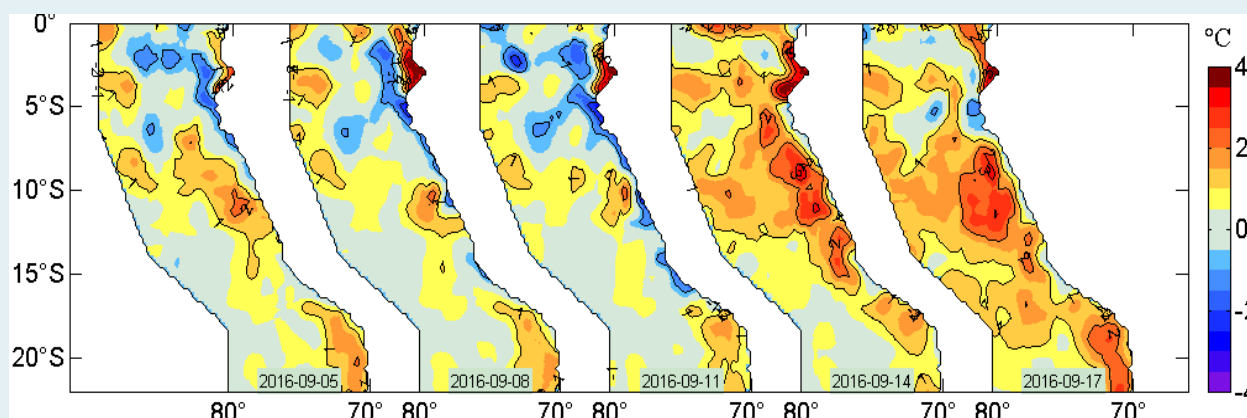
Figura 2. Anomalías de la temperatura superficial del agua (°C) en el mar peruano, cada tres días, entre el 05 y 17 de setiembre del 2016. Datos: AVHRR Global Reyn_SmithOlv2R (Reynolds, et. al., 2007) de CMB/EMC/NCEP de la NOAA. Procesamiento: IMARPE.
