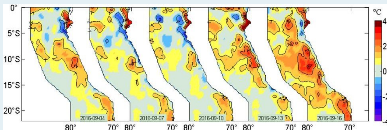
Figura 2. Anomalías de la temperatura superficial del agua (°C) en el mar peruano, cada tres días, entre el 04 y 16 de setiembre del 2016. Datos: AVHRR Global Reyn_SmithOiv2R (Reynolds, et. al., 2007) de CMB/EMC/NCEP de la NOAA. Procesamiento: IMARPE.
