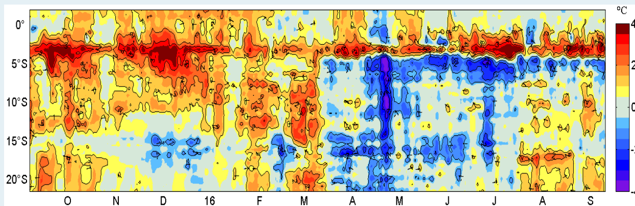
Figura 3. Evolución latitudinal de las anomalías promedio diarias de la temperatura superficial del mar (°C) para la franja de ~50 mn adyacentes al litoral peruano. Datos: AVHRR Global Reyn_SmithOlv2R (Reynolds, et. al., 2007) de CMB/EMC/NCEP de la NOAA. Procesamiento: IMARPE.
