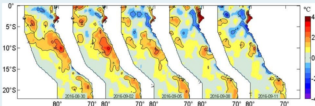
Figura 2. Anomalías de la temperatura superficial del agua (°C) en el mar peruano, cada tres días, entre el 30 de agosto y 11 de setiembre del 2016. Datos: AVHRR Global Reyn_SmithOlv2R (Reynolds, et. al., 2007) de CMB/EMC/NCEP de la NOAA. Procesamiento: IMARPE.
