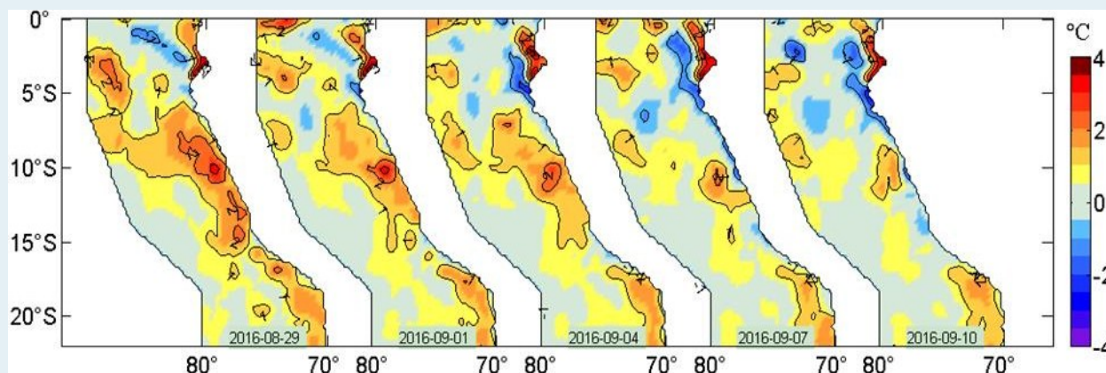
Figura 2. Anomalías de la temperatura superficial del agua (°C) en el mar peruano, cada tres días, entre el 29 de agosto y 10 de setiembre del 2016. Datos: AVHRR Global Reyn_SmithOiv2R (Reynolds, et. al., 2007) de CMB/EMC/NCEP de la NOAA. Procesamiento: IMARPE.
