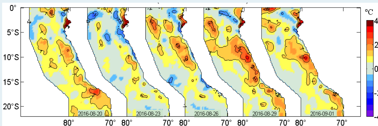
Figura 2. Anomalías de la temperatura superficial del agua (°C) en el mar peruano, cada tres días, entre el 20 de agosto y 01 de setiembre del 2016. Datos: AVHRR Global Reyn_SmithOiv2R (Reynolds, et. al., 2007) de CMB/EMC/NCEP de la NOAA. Procesamiento: IMARPE.
