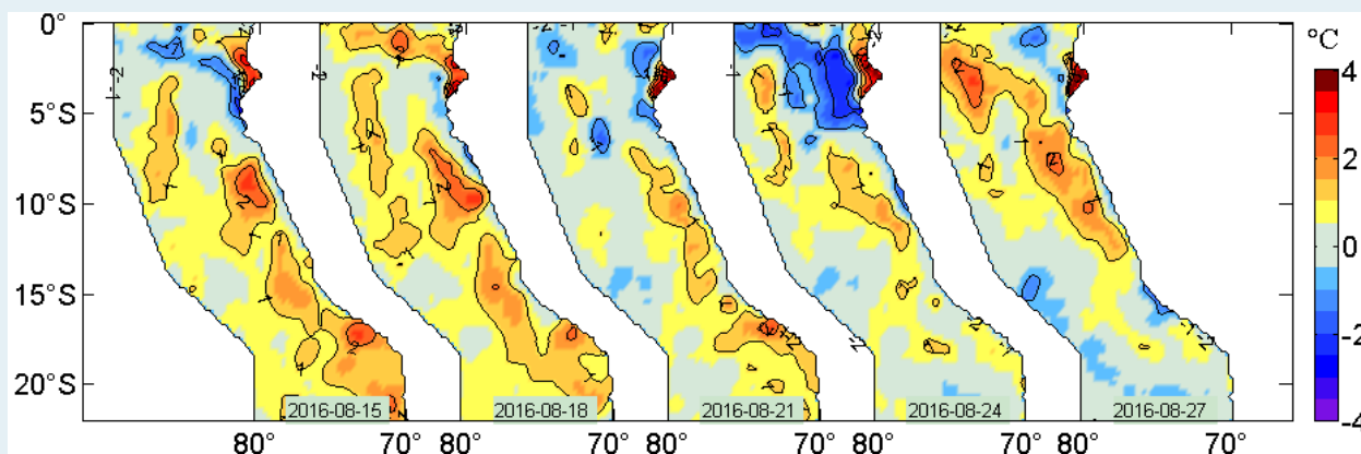
Figura 2. Anomalías de la temperatura superficial del agua (°C) en el mar peruano, cada tres días, entre el 15 y 27 de agosto del 2016. Datos: AVHRR Global Reyn_SmithOiv2R (Reynolds, et. al., 2007) de CMB/EMC/NCEP de la NOAA. Procesamiento: IMARPE.
