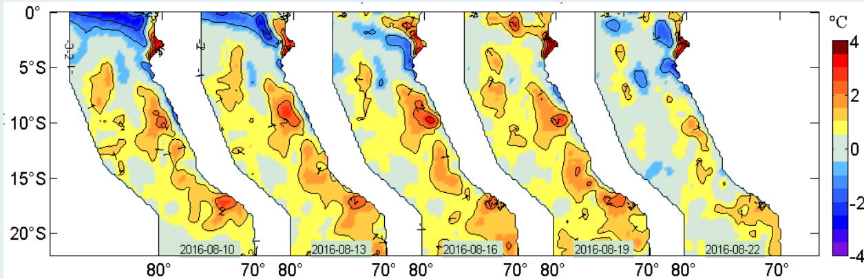
Figura 2. Anomalías de la temperatura superficial del agua (°C) en el mar peruano, cada tres días, entre el 10 y 22 de agosto del 2016. Datos: AVHRR Global Reyn_SmithOiv2R (Reynolds, et. al., 2007) de CMB/EMC/NCEP de la NOAA. Procesamiento: IMARPE.
