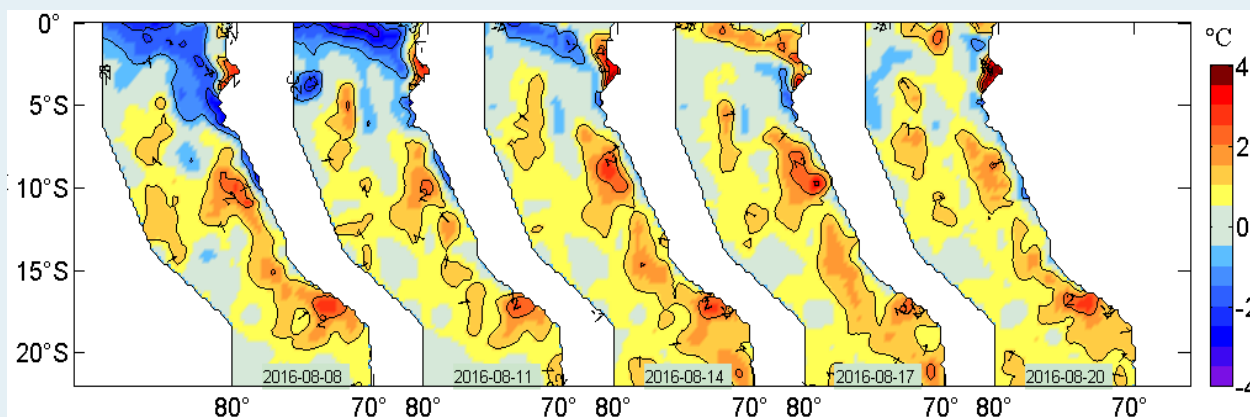
Figura 2. Anomalías de la temperatura superficial del agua (°C) en el mar peruano, cada tres días, entre el 08 y 20 de agosto del 2016. Datos: AVHRR Global Reyn_SmithOiv2R (Reynolds, et. al., 2007) de CMB/EMC/NCEP de la NOAA. Procesamiento: IMARPE.
