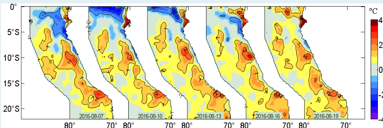
Figura 2. Anomalías de la temperatura superficial del agua (°C) en el mar peruano, cada tres días, entre el 07 y 19 de agosto del 2016. Datos: AVHRR Global Reyn_SmithOIv2R (Reynolds, et. al., 2007) de CMB/EMC/NCEP de la NOAA. Procesamiento: IMARPE.
