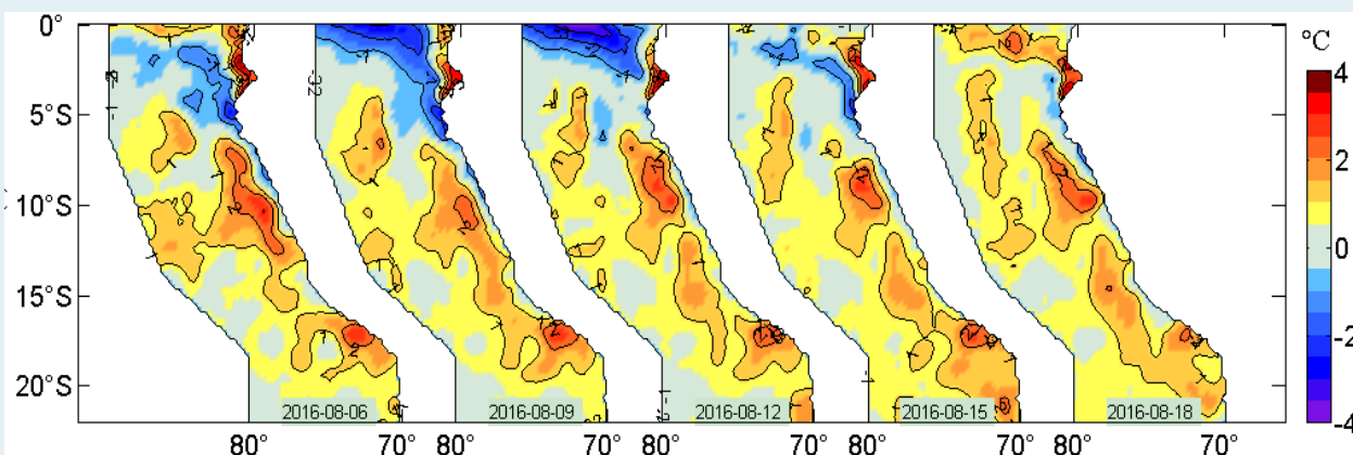
Figura 2. Anomalías de la temperatura superficial del agua (°C) en el mar peruano, cada tres días, entre el 06 y 18 de agosto del 2016. Datos: AVHRR Global Reyn_SmithOiv2R (Reynolds, et. al., 2007) de CMB/EMC/NCEP de la NOAA. Procesamiento: IMARPE.
