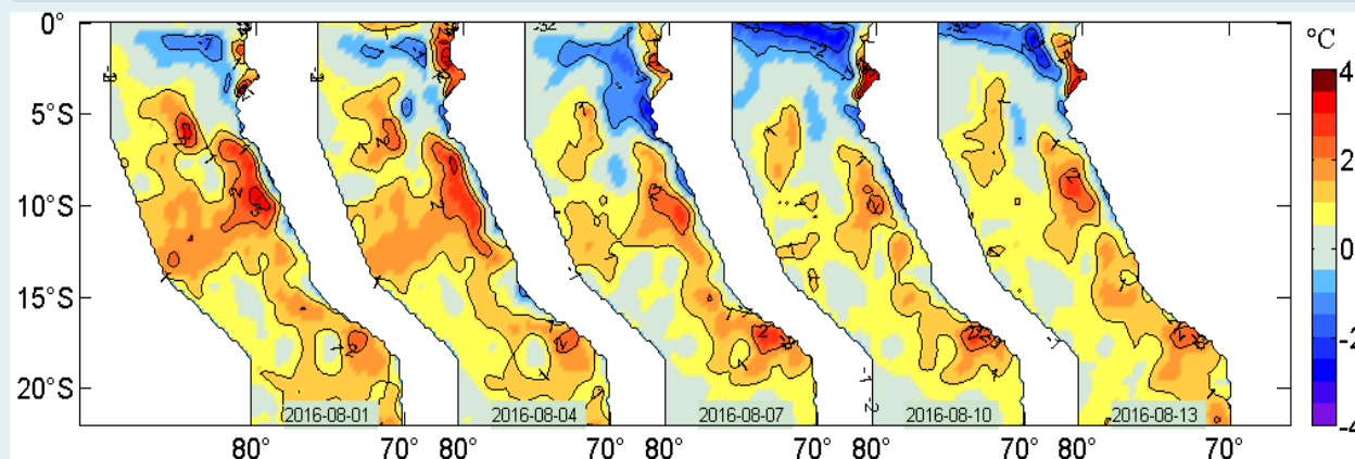
Figura 2. Anomalías de la temperatura superficial del agua (°C) en el mar peruano, cada tres días, entre el 01 y 13 de agosto del 2016. Datos: AVHRR Global Reyn_SmithOiv2R (Reynolds, et. al., 2007) de CMB/EMC/NCEP de la NOAA. Procesamiento: IMARPE.
