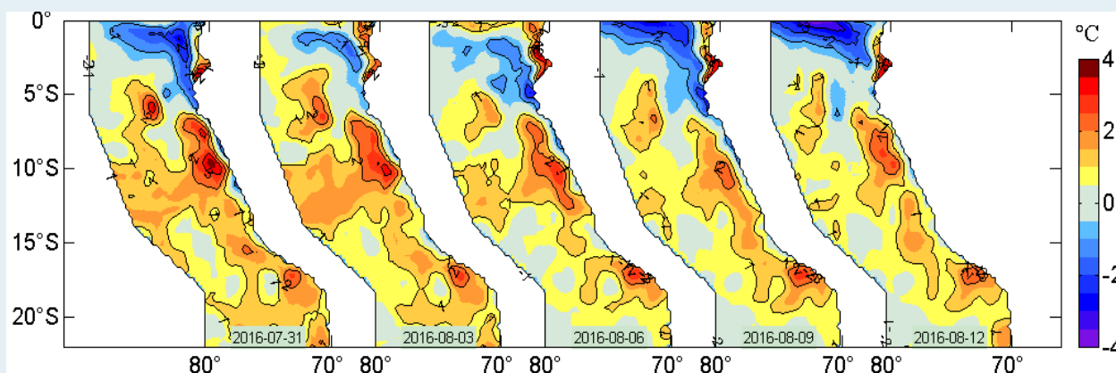
Figura 2. Anomalías de la temperatura superficial del agua (°C) en el mar peruano, cada tres días, entre el 31 de julio y 12 de agosto del 2016. Datos: AVHRR Global Reyn_SmithOiv2R (Reynolds, et. al., 2007) de CMB/EMC/NCEP de la NOAA. Procesamiento: IMARPE.
