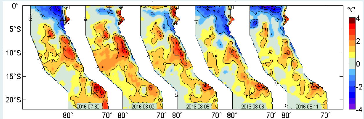
Figura 2. Anomalías de la temperatura superficial del agua (°C) en el mar peruano, cada tres días, entre el 30 de julio y 11 de agosto del 2016. Datos: AVHRR Global Reyn_SmithOlv2R (Reynolds, et. al., 2007) de CMB/EMC/NCEP de la NOAA. Procesamiento: IMARPE.
