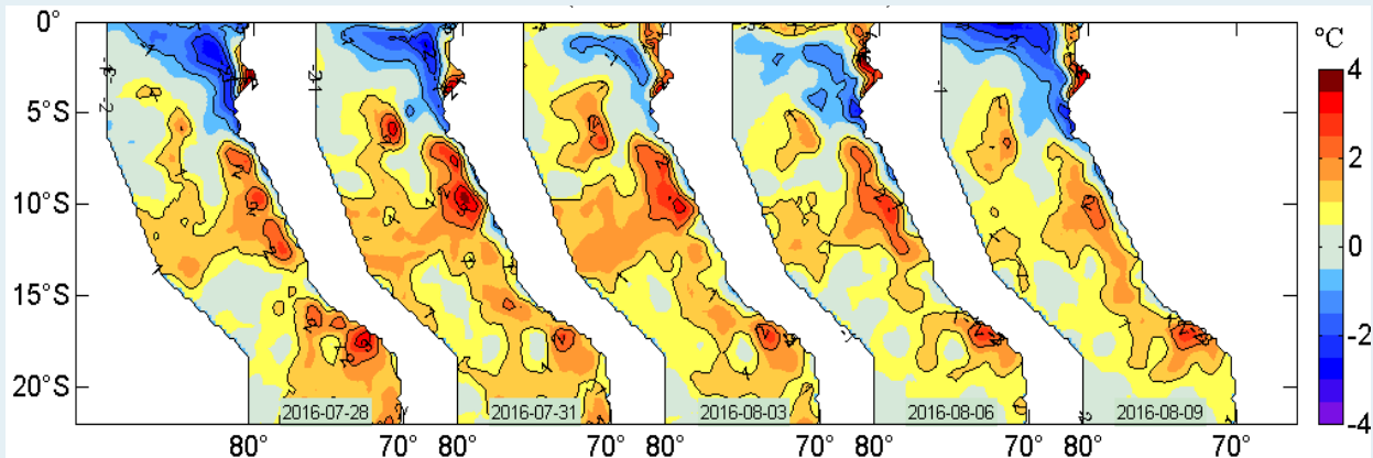
Figura 2. Anomalías de la temperatura superficial del agua (°C) en el mar peruano, cada tres días, entre el 28 de julio y 09 de agosto del 2016. Datos: AVHRR Global Reyn_SmithOlv2R (Reynolds, et. al., 2007) de CMB/EMC/NCEP de la NOAA. Procesamiento: IMARPE.
