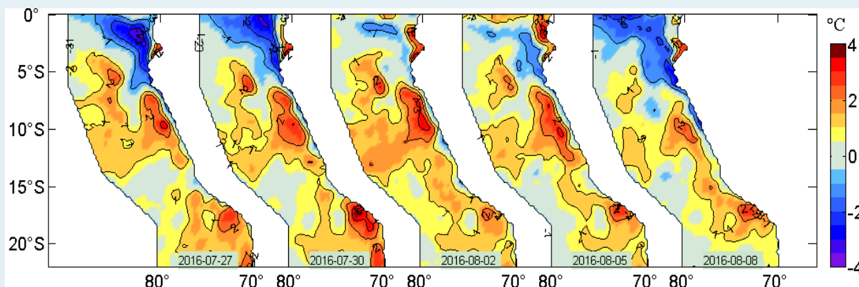
Figura 2. Anomalías de la temperatura superficial del agua (°C) en el mar peruano, cada tres días, entre el 27 de julio y 08 de agosto del 2016. Datos: AVHRR Global Reyn_SmithOiv2R (Reynolds, et. al., 2007) de CMB/EMC/NCEP de la NOAA. Procesamiento: IMARPE.
