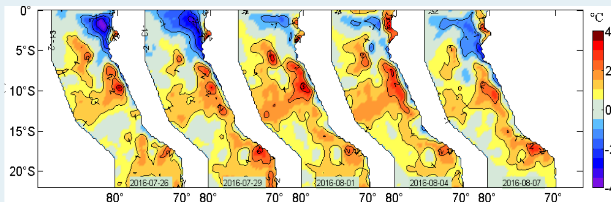
Figura 2. Anomalías de la temperatura superficial del agua (°C) en el mar peruano, cada tres días, entre el 26 de julio y 07 de agosto del 2016. Datos: AVHRR Global Reyn_SmithOiv2R (Reynolds, et. al., 2007) de CMB/EMC/NCEP de la NOAA. Procesamiento: IMARPE.
