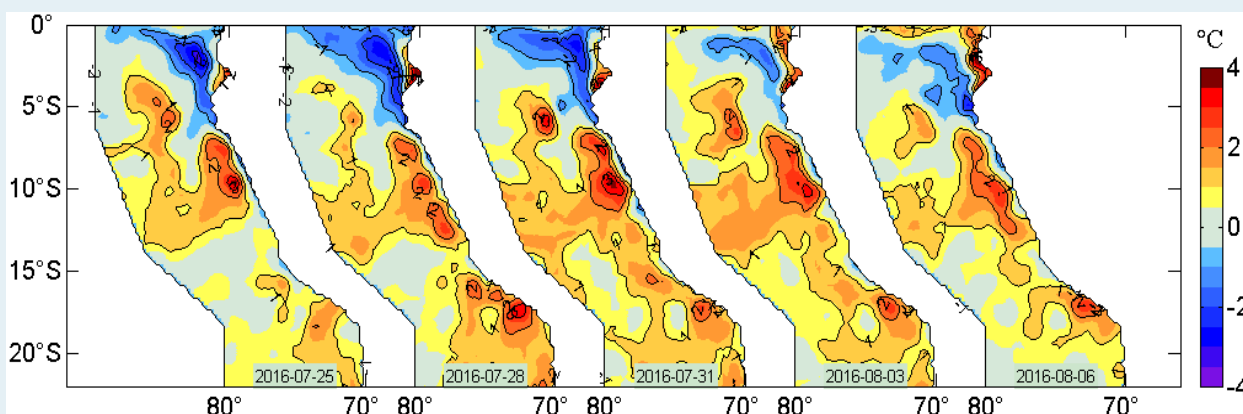
Figura 2. Anomalías de la temperatura superficial del agua (°C) en el mar peruano, cada tres días, entre el 25 de julio y 06 de agosto del 2016. Datos: AVHRR Global Reyn_SmithOlv2R (Reynolds, et. al., 2007) de CMB/EMC/NCEP de la NOAA. Procesamiento: IMARPE.
