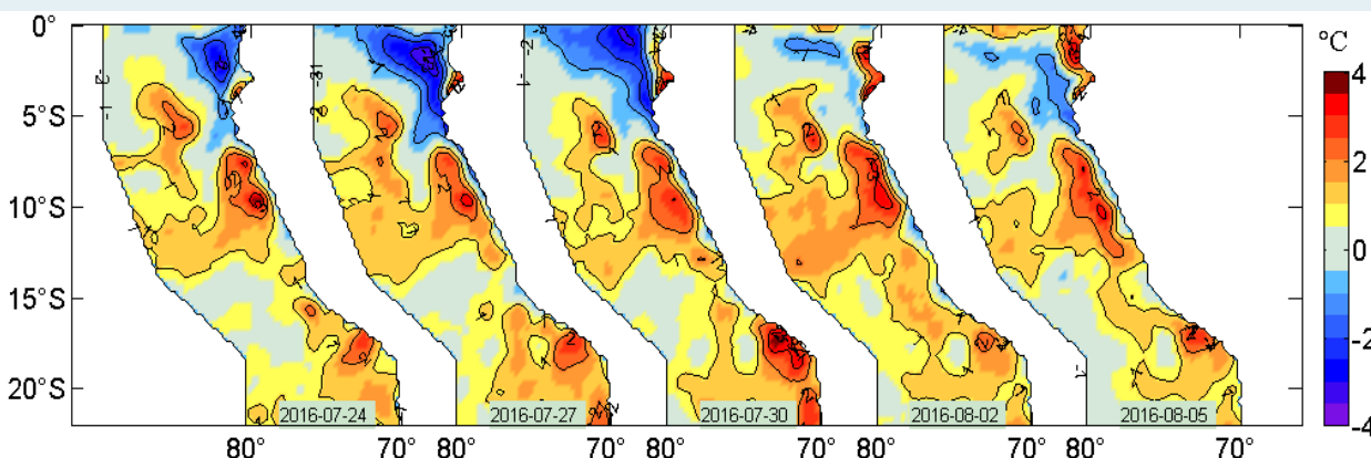
Figura 2. Anomalías de la temperatura superficial del agua (°C) en el mar peruano, cada tres días, entre el 24 de julio y 05 de agosto del 2016. Datos: AVHRR Global Reyn_SmithOlv2R (Reynolds, et. al., 2007) de CMB/EMC/NCEP de la NOAA. Procesamiento: IMARPE.
