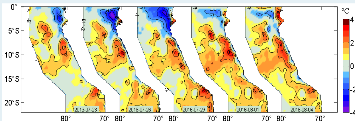
Figura 2. Anomalías de la temperatura superficial del agua (°C) en el mar peruano, cada tres días, entre el 23 de julio y 04 de agosto del 2016. Datos: AVHRR Global Reyn_SmithOIv2R (Reynolds, et. al., 2007) de CMB/EMC/NCEP de la NOAA. Procesamiento: IMARPE.
