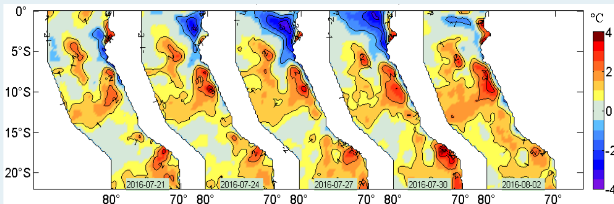
Figura 2. Anomalías de la temperatura superficial del agua (°C) en el mar peruano, cada tres días, entre el 21 de julio y 02 de agosto del 2016. Datos: AVHRR Global Reyn_SmithOIv2R (Reynolds, et. al., 2007) de CMB/EMC/NCEP de la NOAA. Procesamiento: IMARPE.
