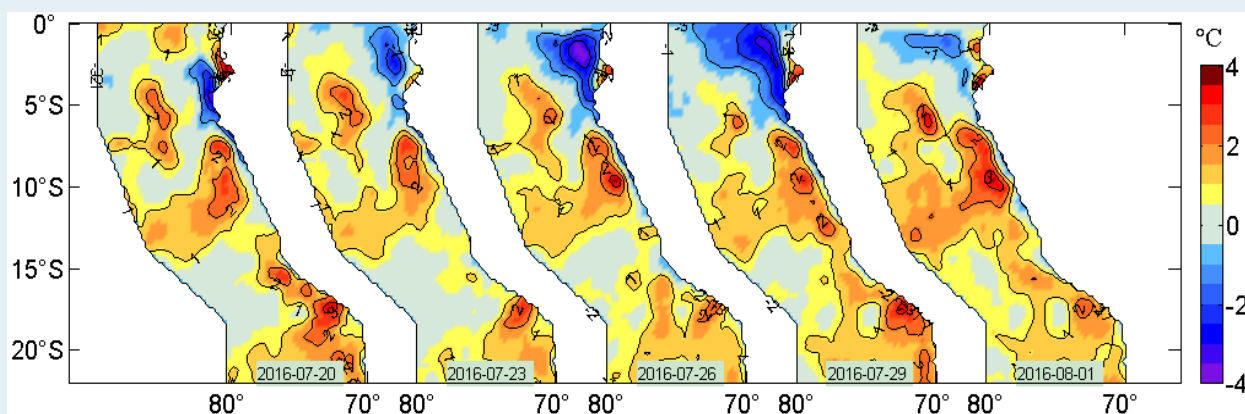
Figura 2. Anomalías de la temperatura superficial del agua (°C) en el mar peruano, cada tres días, entre el 20 de julio y 01 de agosto del 2016. Datos: AVHRR Global Reyn_SmithOiv2R (Reynolds, et. al., 2007) de CMB/EMC/NCEP de la NOAA. Procesamiento: IMARPE.
