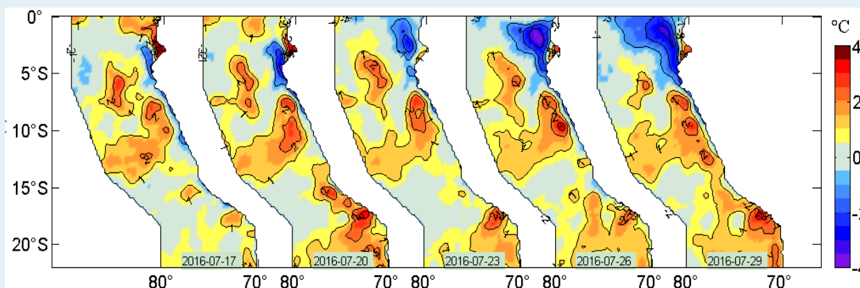
Figura 2. Anomalías de la temperatura superficial del agua (°C) en el mar peruano, cada tres días, entre el 17 y 29 de julio del 2016. Datos: AVHRR Global Reyn_SmithOlv2R (Reynolds, et. al., 2007) de CMB/EMC/NCEP de la NOAA. Procesamiento: IMARPE.
