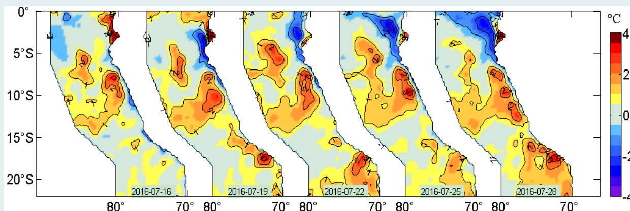
Figura 2. Anomalías de la temperatura superficial del agua (°C) en el mar peruano, cada tres días, entre el 16 y 28 de julio del 2016. Datos: AVHRR Global Reyn_SmithO1v2R (Reynolds, et. al., 2007) de CMB/EMC/NCEP de la NOAA. Procesamiento: IMARPE.
