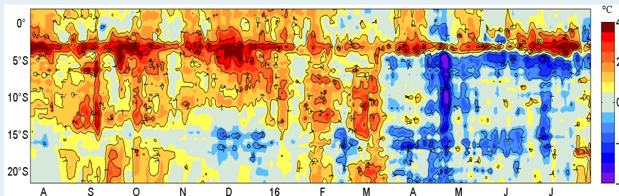
Figura 3. Evolución latitudinal de las anomalías promedio diarias de la temperatura superficial del mar (°C) para la franja de ~50 mn adyacentes al litoral peruano. Datos: AVHRR Global Reyn_SmithO1v2R (Reynolds, et. al., 2007) de CMB/EMC/NCEP de la NOAA. Procesamiento: IMARPE.
