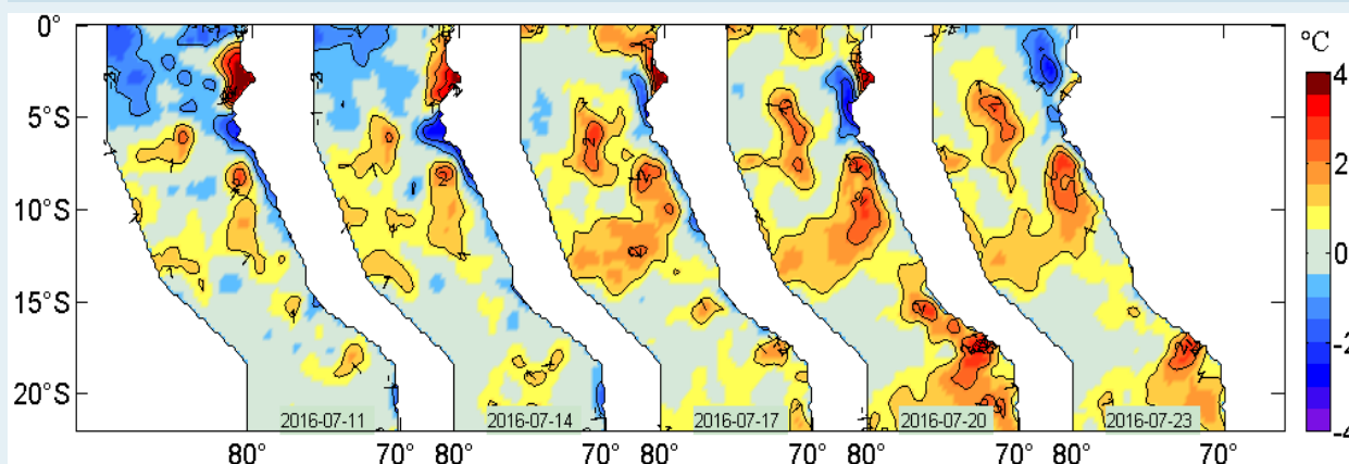
Figura 2. Anomalías de la temperatura superficial del agua (°C) en el mar peruano, cada tres días, entre el 11 y 23 de julio del 2016. Datos: AVHRR Global Reyn_SmithOIv2R (Reynolds, et. al., 2007) de CMB/EMC/NCEP de la NOAA. Procesamiento: IMARPE.
