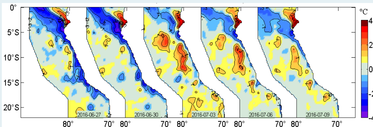
Figura 2. Anomalías de la temperatura superficial del agua (°C) en el mar peruano, cada tres días, entre el 27 de junio y 09 de julio del 2016. Datos: AVHRR Global Reyn_SmithOiv2R (Reynolds, et. al., 2007) de CMB/EMC/NCEP de la NOAA. Procesamiento: IMARPE.
