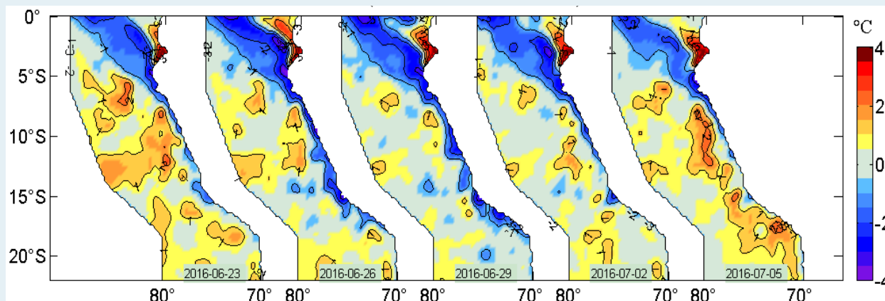
Figura 2. Anomalías de la temperatura superficial del agua (°C) en el mar peruano, cada tres días, entre el 23 de junio y 05 de julio del 2016. Datos: AVHRR Global Reyn_SmithOiv2R (Reynolds, et. al., 2007) de CMB/EMC/NCEP de la NOAA. Procesamiento: IMARPE.
