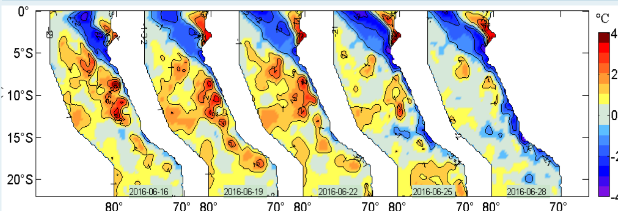
Figura 2. Anomalías de la temperatura superficial del agua (°C) en el mar peruano, cada tres días, entre el 16 y 28 de junio del 2016. Datos: AVHRR Global Reyn_SmithOiv2R (Reynolds, et. al., 2007) de CMB/EMC/NCEP de la NOAA. Procesamiento: IMARPE.
