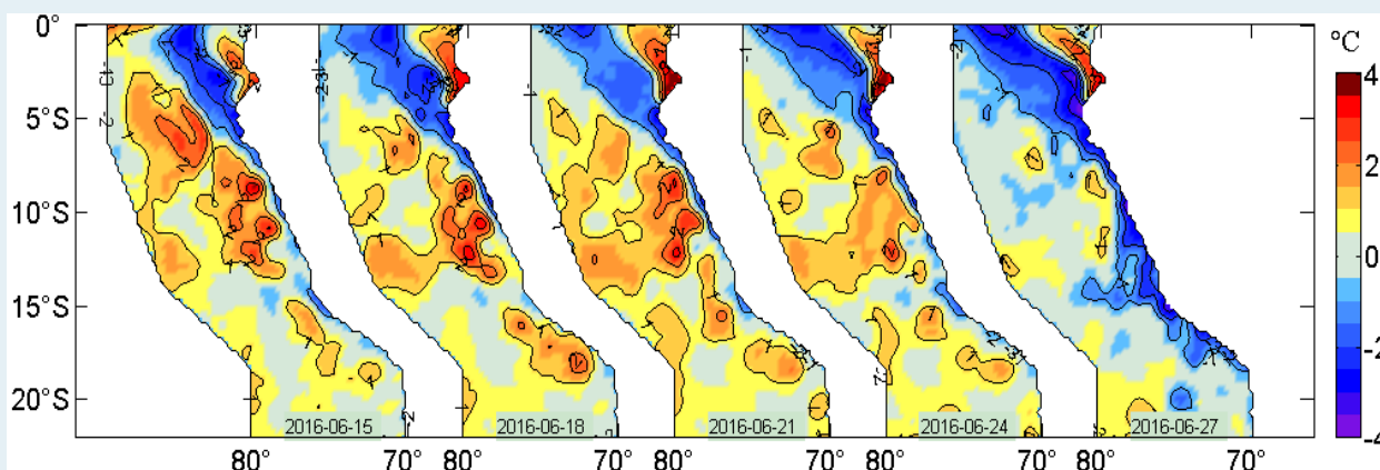
Figura 2. Anomalías de la temperatura superficial del agua (°C) en el mar peruano, cada tres días, entre el 15 y 27 de junio del 2016. Datos: AVHRR Global Reyn_SmithOiv2R (Reynolds, et. al., 2007) de CMB/EMC/NCEP de la NOAA. Procesamiento: IMARPE.
