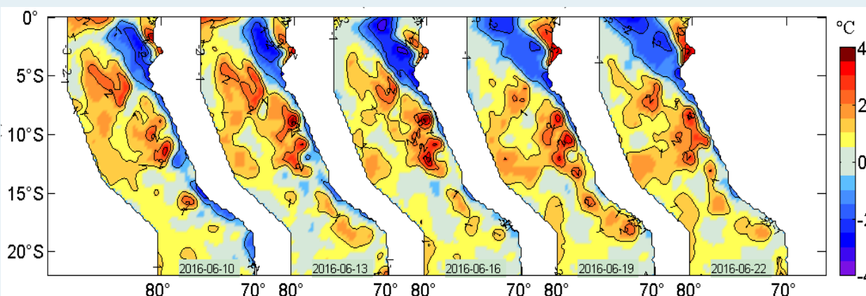
Figura 2. Anomalías de la temperatura superficial del agua (°C) en el mar peruano, cada tres días, entre el 10 y 22 de junio del 2016. Datos: AVHRR Global Reyn_SmithOiv2R (Reynolds, et. al., 2007) de CMB/EMC/NCEP de la NOAA. Procesamiento: IMARPE.
