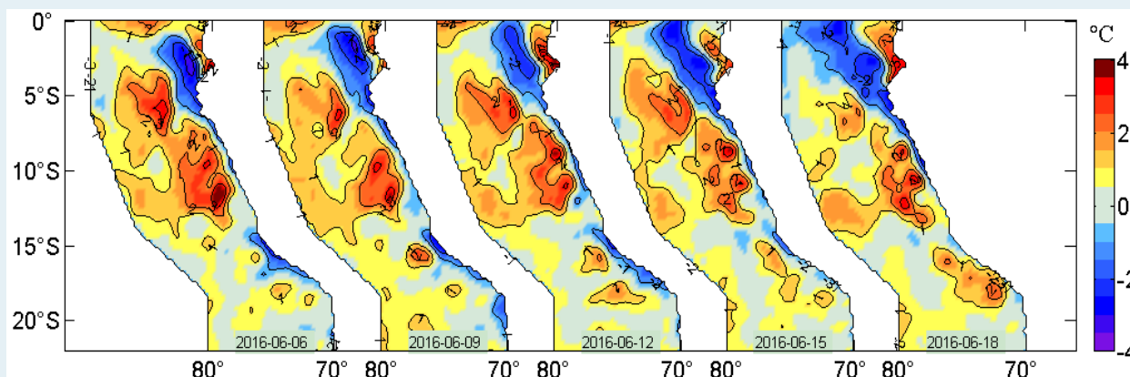
Figura 2. Anomalías de la temperatura superficial del agua (°C) en el mar peruano, cada tres días, entre el 06 y 18 de junio del 2016. Datos: AVHRR Global Reyn_SmithOlv2R (Reynolds, et. al., 2007) de CMB/EMC/NCEP de la NOAA. Procesamiento: IMARPE.
