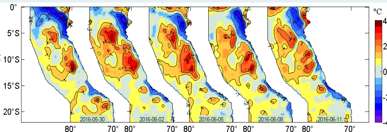
Figura 2. Anomalías de la temperatura superficial del agua (°C) en el mar peruano, cada tres días, entre el 30 de mayo y 11 de junio del 2016. Datos: AVHRR Global Reyn_SmithOiv2R (Reynolds, et. al., 2007) de CMB/EMC/NCEP de la NOAA. Procesamiento: IMARPE.
