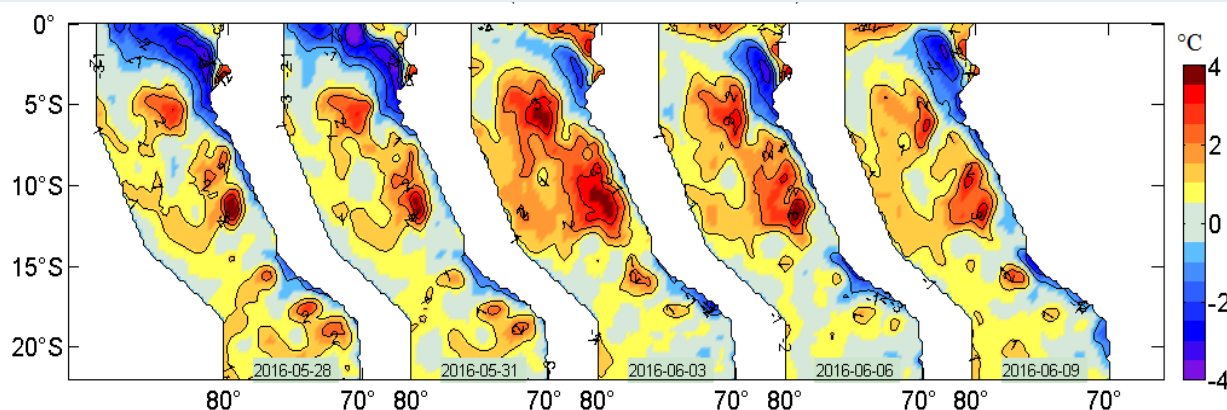
Figura 2. Anomalías de la temperatura superficial del agua (°C) en el mar peruano, cada tres días, entre el 28 de mayo y 09 de junio del 2016. Datos: AVHRR Global Reyn_SmithOIv2R (Reynolds, et. al., 2007) de CMB/EMC/NCEP de la NOAA. Procesamiento: IMARPE.
