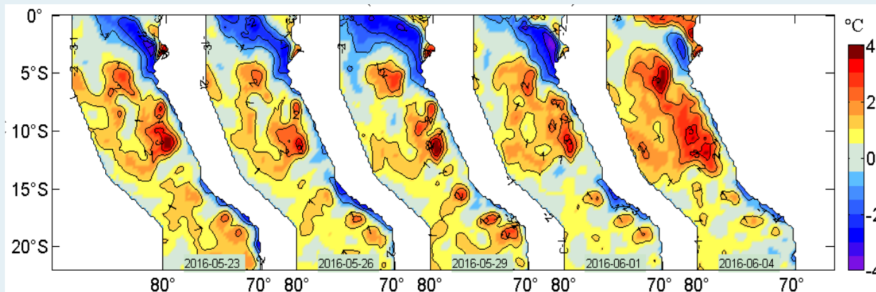
Figura 2. Anomalías de la temperatura superficial del agua (°C) en el mar peruano, cada tres días, entre el 23 de mayo y 04 de junio del 2016. Datos: AVHRR Global Reyn_SmithOlv2R (Reynolds, et. al., 2007) de CMB/EMC/NCEP de la Administración Nacional del Océano y la Atmósfera (NOAA, según sus siglas en inglés). Procesamiento: IMARPE.
