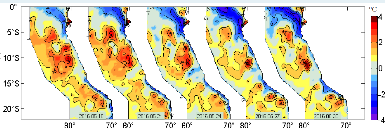
Figura 2. Anomalías de la temperatura superficial del agua (°C) en el mar peruano, cada tres días, entre el 18 y 30 de mayo del 2016. Datos: AVHRR Global Reyn_SmithOiv2R (Reynolds, et. al., 2007) de CMB/EMC/NCEP de la NOAA. Procesamiento: IMARPE.
