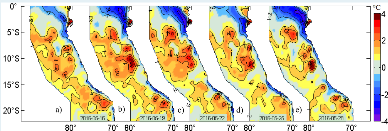
Figura 2. Anomalías de la temperatura superficial del agua (°C) en el mar peruano, cada tres días, entre el 16 y 28 de mayo del 2016. Datos: AVHRR Global Reyn_SmithOiv2R (Reynolds, et. al., 2007) de CMB/EMC/NCEP de la NOAA, según sus siglas en inglés. Procesamiento: IMARPE.
