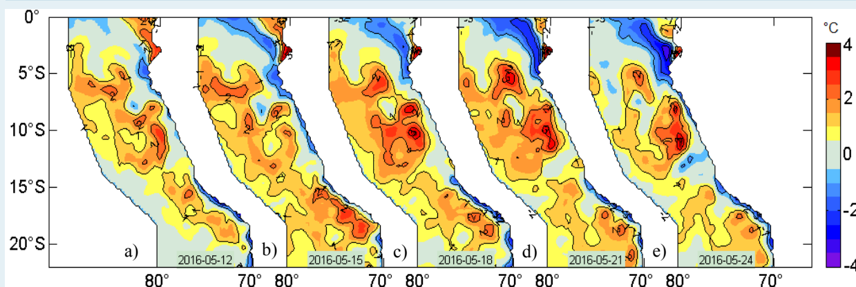
Figura 2. Anomalías de la temperatura superficial del agua (°C) en el mar peruano, cada tres días, entre el 12 y 24 de mayo del 2016. Datos: AVHRR Global Reyn_SmithOiv2R (Reynolds, et. al., 2007) de CMB/EMC/NCEP de la NOAA. Procesamiento: IMARPE.
